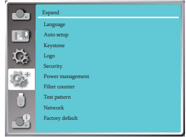
확장메뉴 화면
